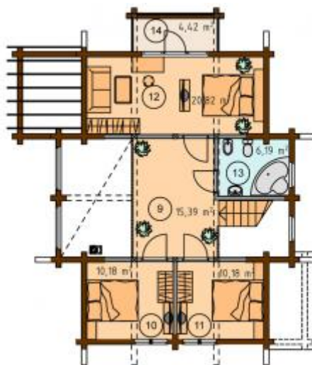
2 этаж Общая площадь: 67,19 м 2 Площадь помещений: 62,78 м 2
